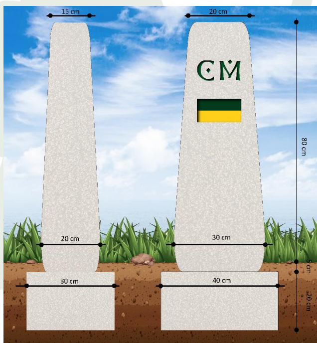
Modello D. 1 Cippo in cemento precompresso. Segnaletica extraurbana.
